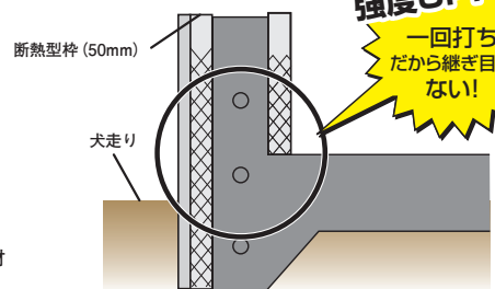
タイト・モールド 基礎断面図
