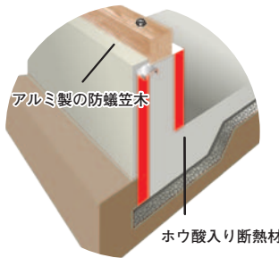
タイト・モールド 基礎断面図
